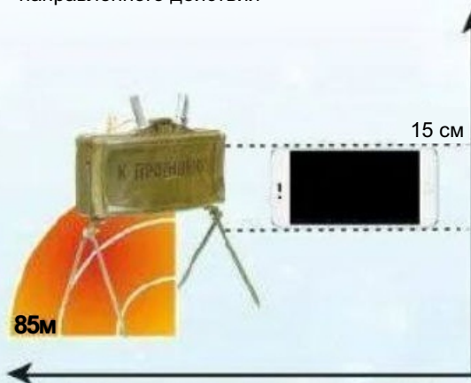
«МОН-50» - противопехотная мина направленного действия
